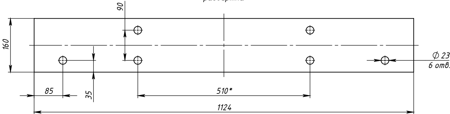
Поз.1 (Полухомут) развертка
