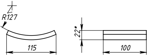
Поз.2 (Упор) 1: 5
